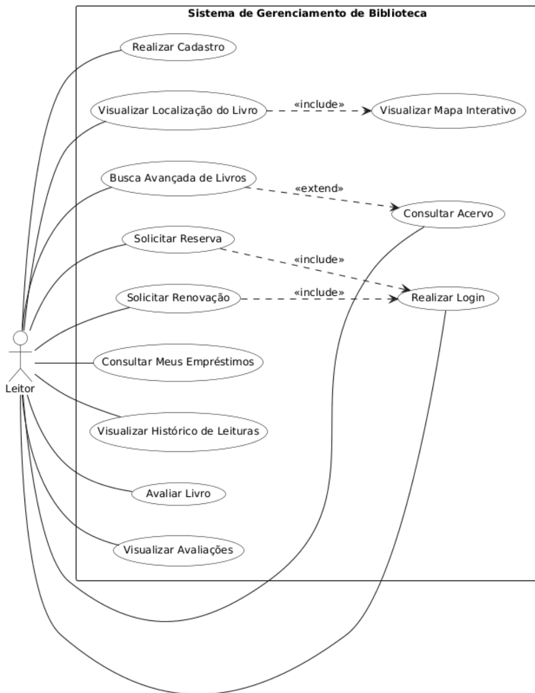
Figura 2 – Diagrama de Casos de Uso: Módulo Leitor
